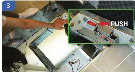
사다리 고정 장치를 눌러 사다리 펼치기
